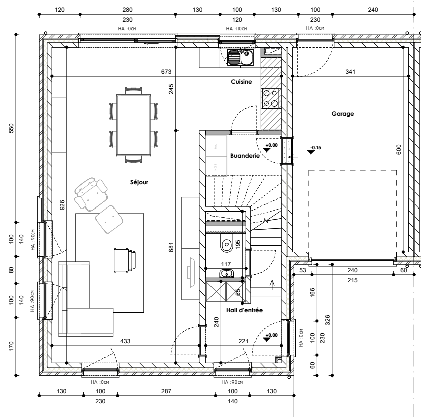
Rez-de-chaussée
