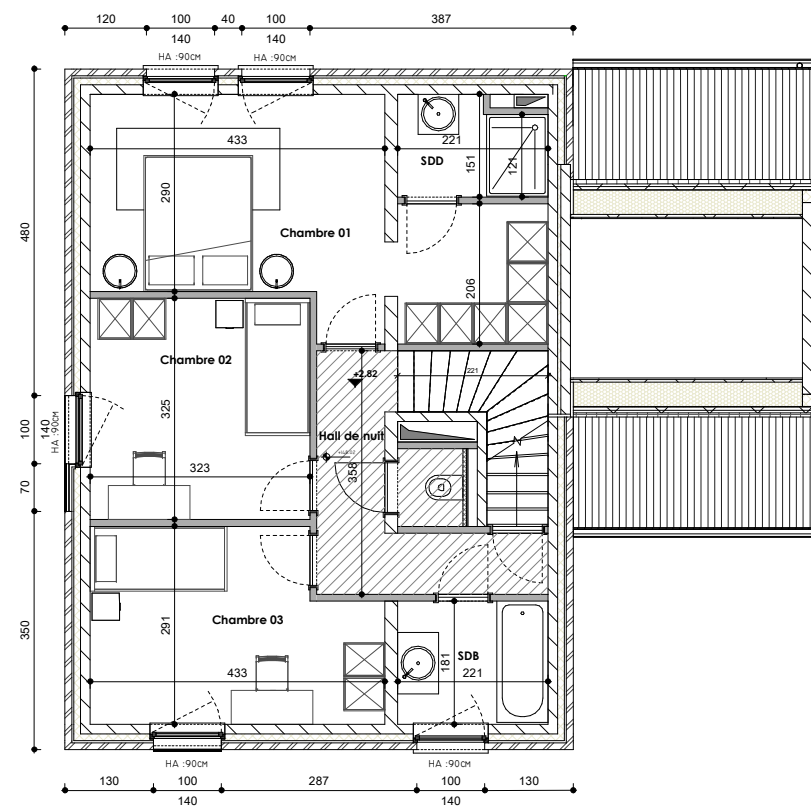
Premier étage
