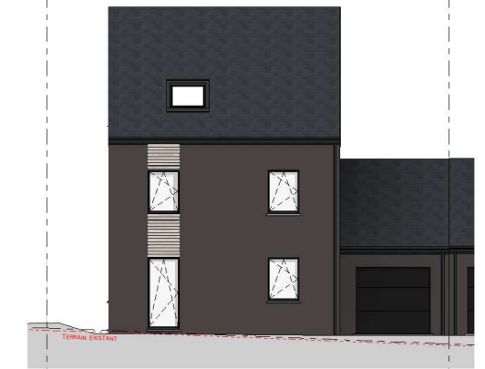
Elévation rue
