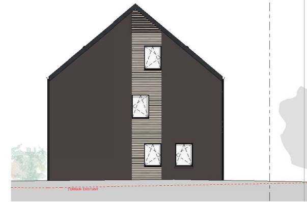
Elévation jardin
